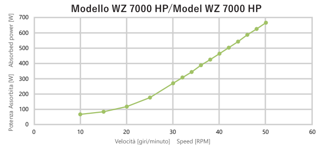
Grafico velocità / Potenza assorbita Graph Speed [RPM] vs Absorbed power [W]
